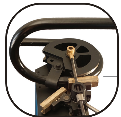
Matrice con rotazione dx/sx (opzionale) Former L/E bending (optional)
